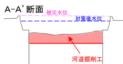
【断面図】
