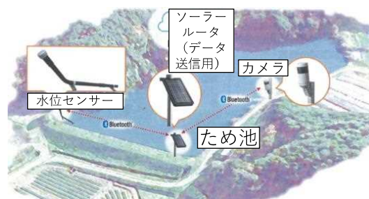
ため池の監視システム概要図
