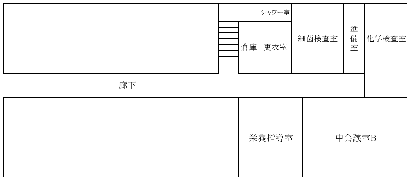
1階 平面図
