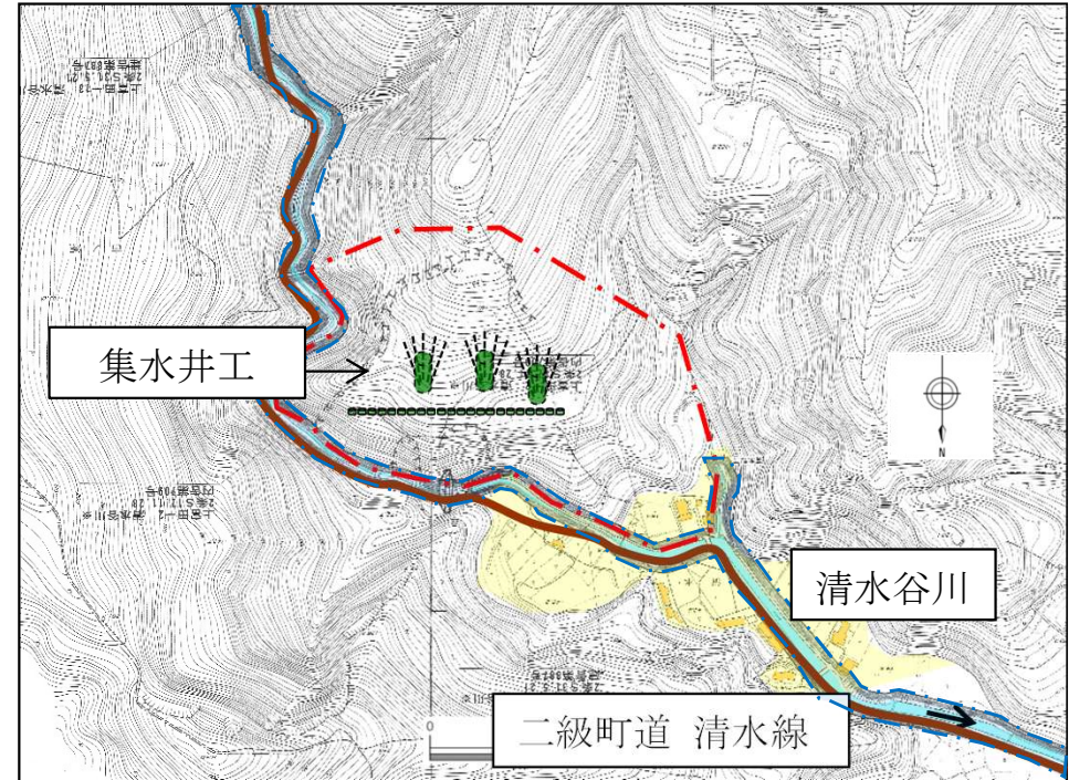
地すべり対策施設の整備
