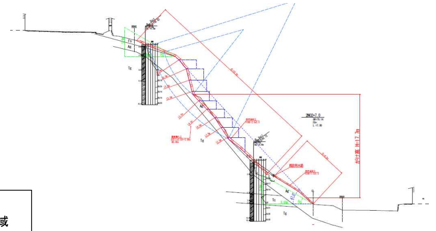
横断図
