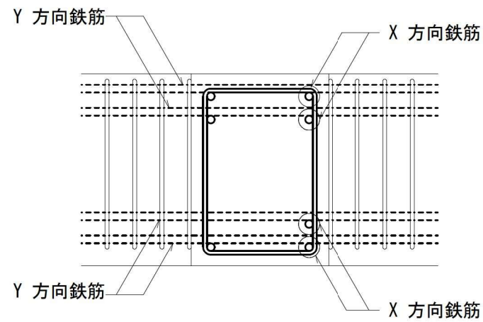
梁主筋上下関係
