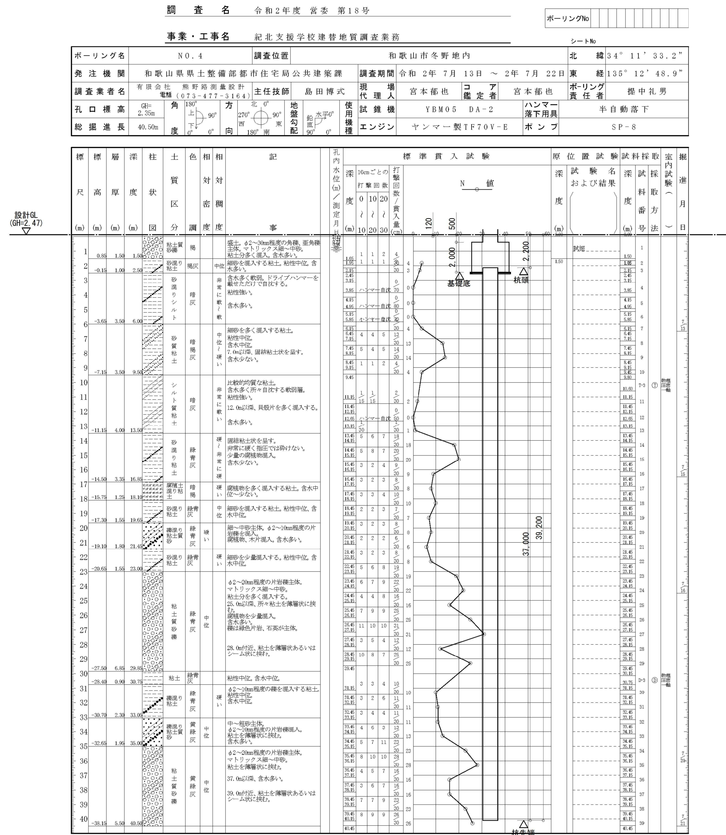
ボーリング柱状図
