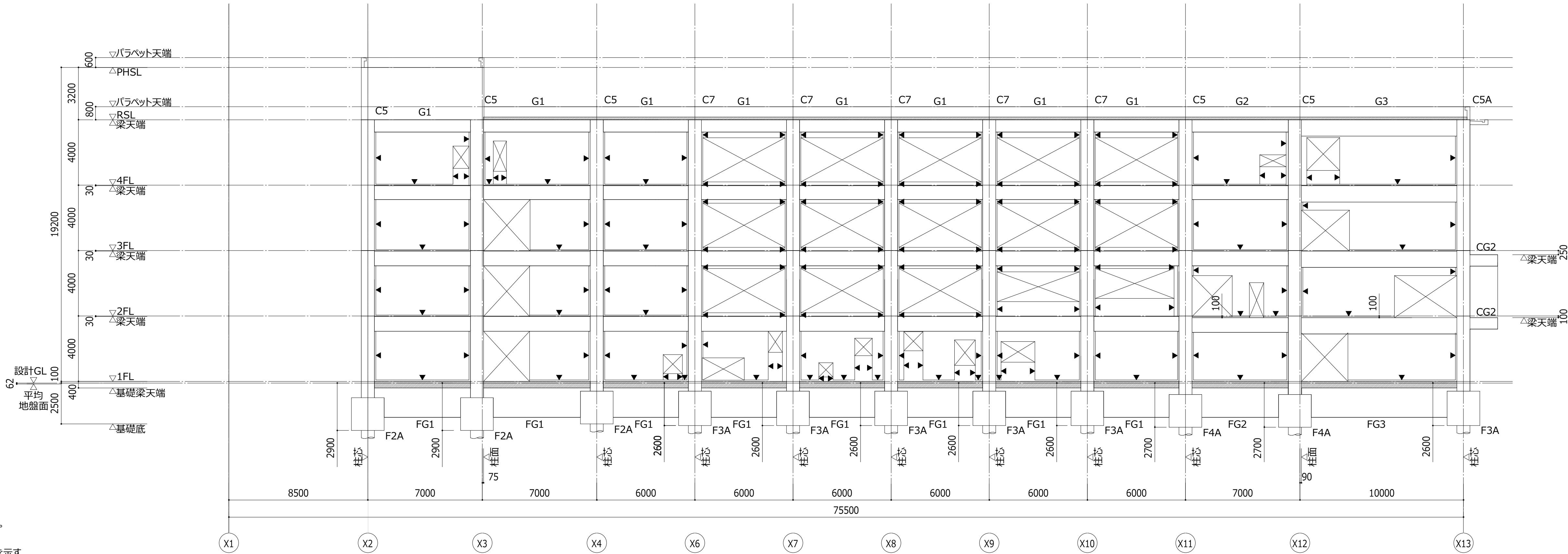
Y14 通り軸組図 1/150 [A1] 1/300 [A3]
