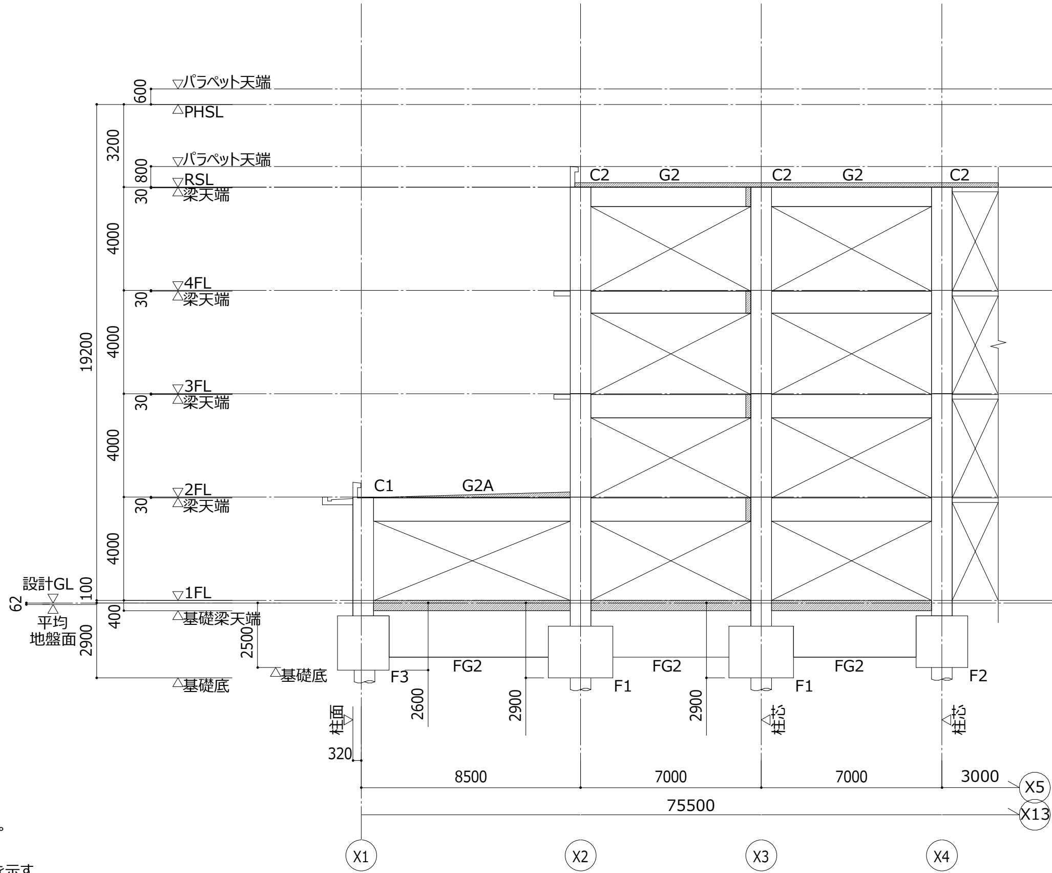
Y11 通り軸組図 1/150 [A1] 1/300 [A3]
