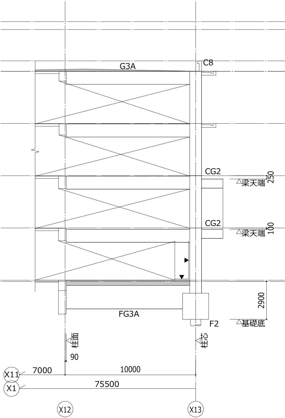
Y12 通り軸組図 1/150 [A1] 1/300 [A3]
