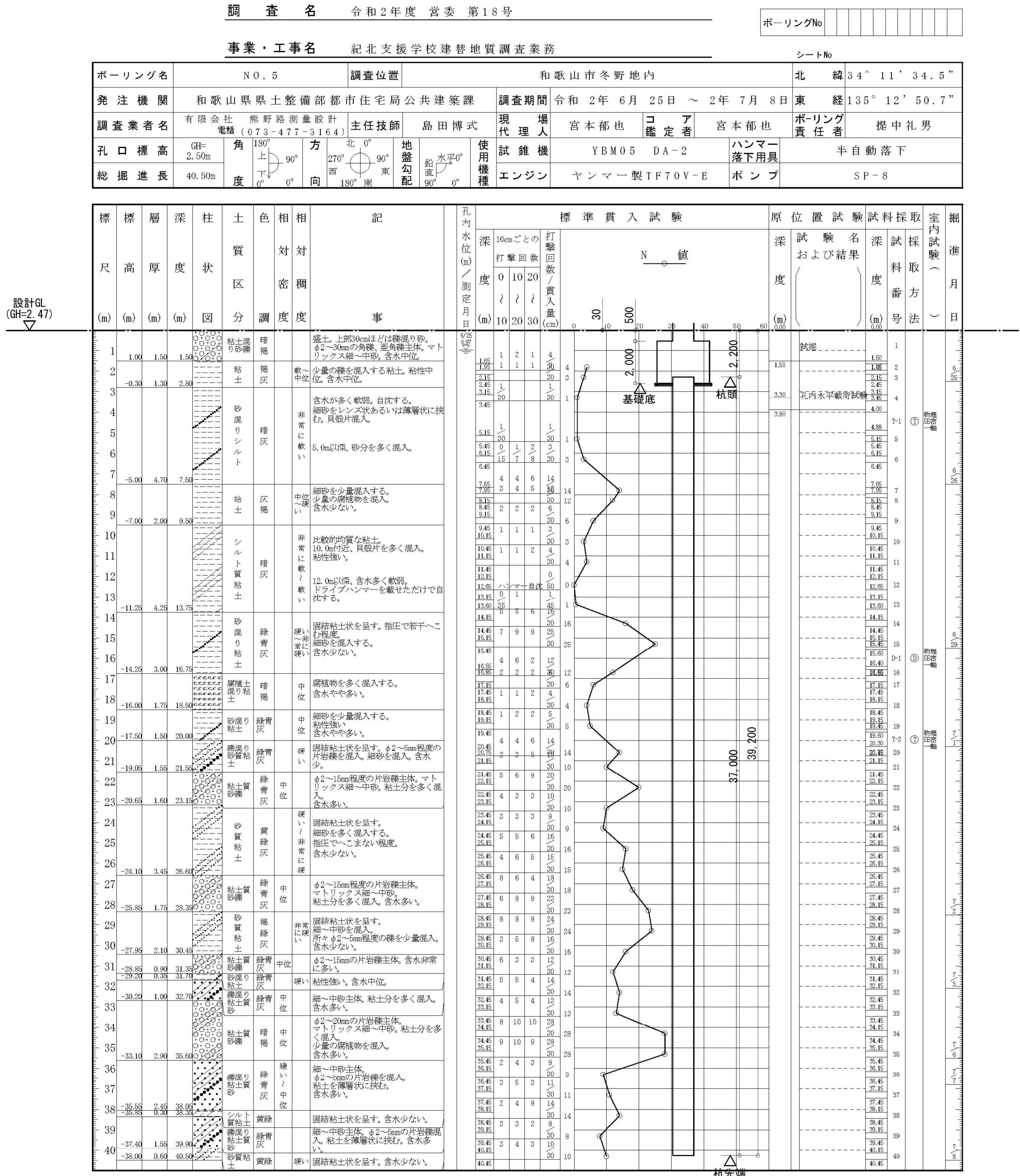
ボーリング柱状図
