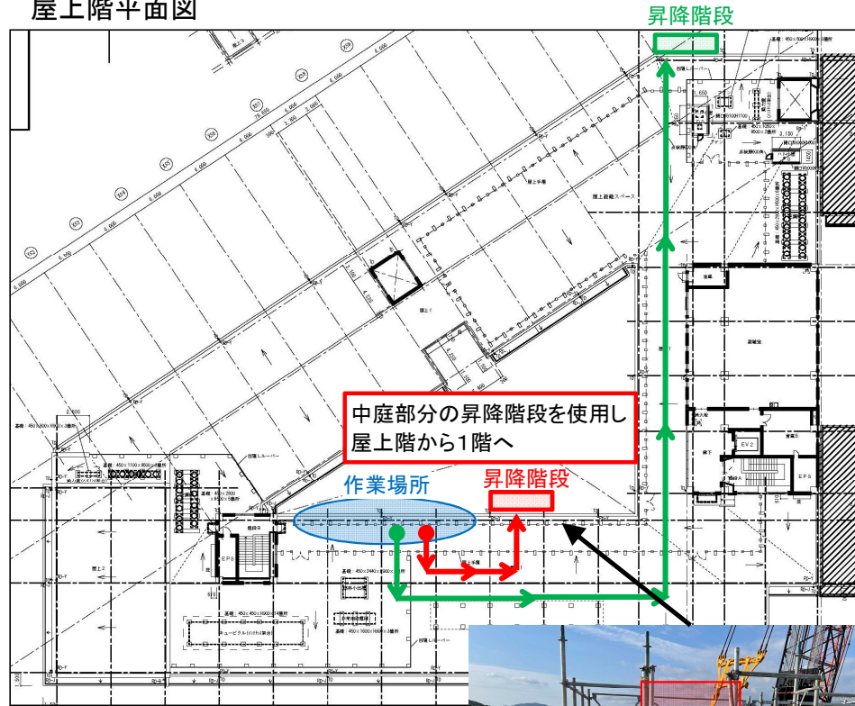
屋上階平面図
