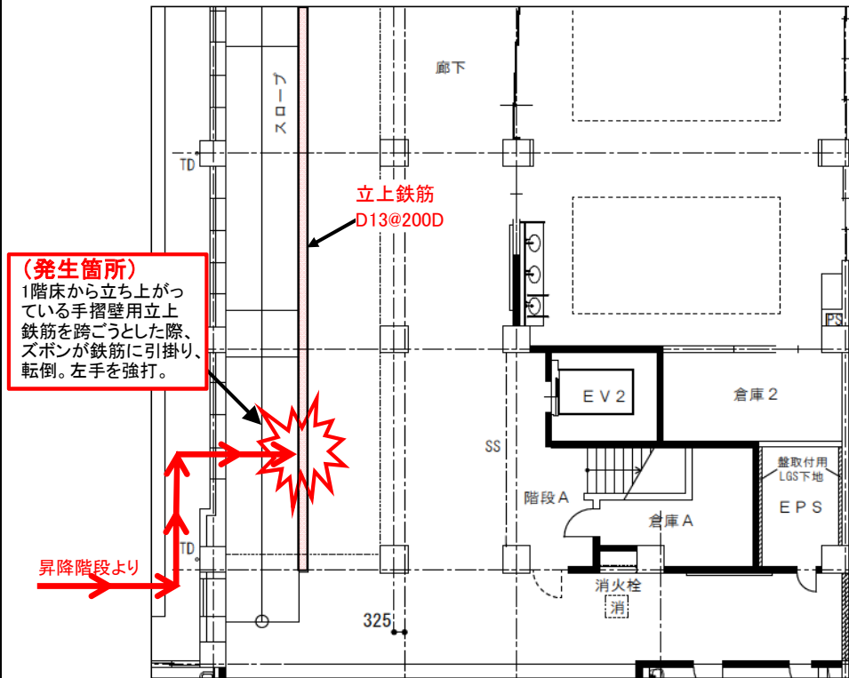
1階発生箇所平面図
