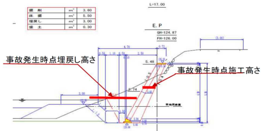
断面図
