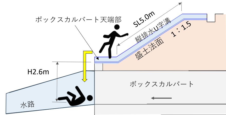
断面図（縦排水溝部）
