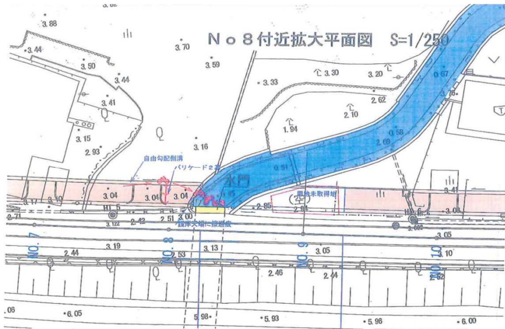
平面図
