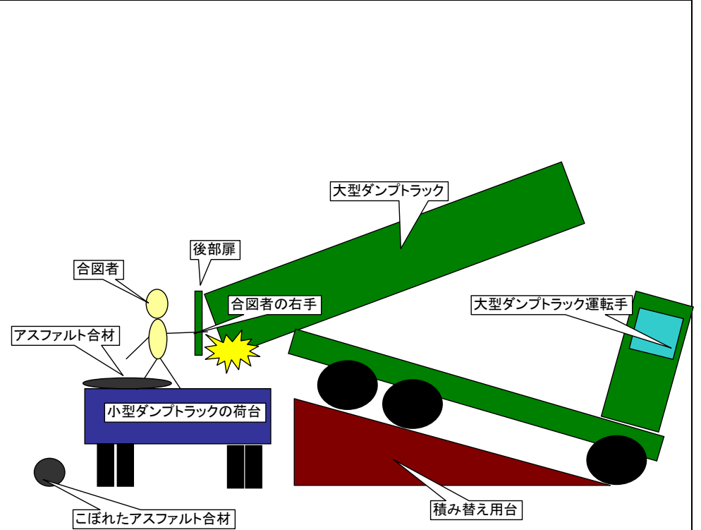
事故状況断面図
