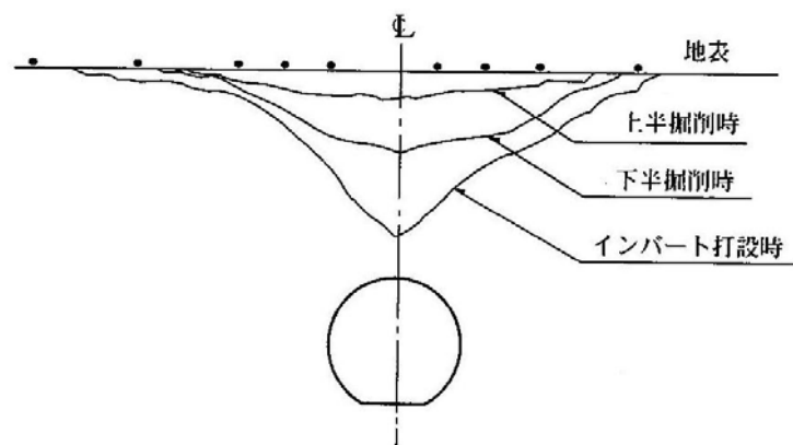
図 6 - 13 地表沈下分布
