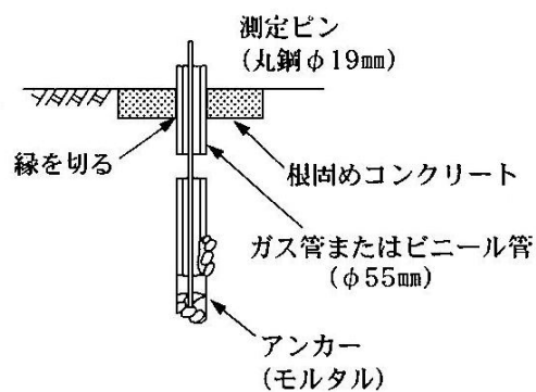
図 6 - 8 地中沈下測定点 of 設置例
