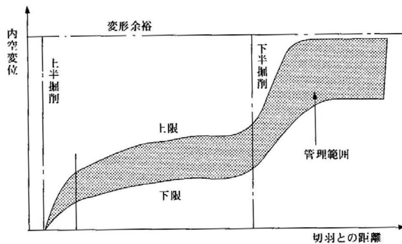
図 5 - 4 内空変位管理図の例
