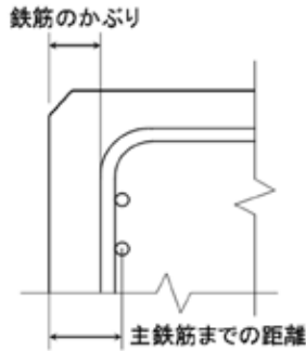
図1-3-1 鉄筋のかぶり
