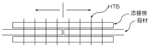
図3-2-1 ボルト締付け順序
