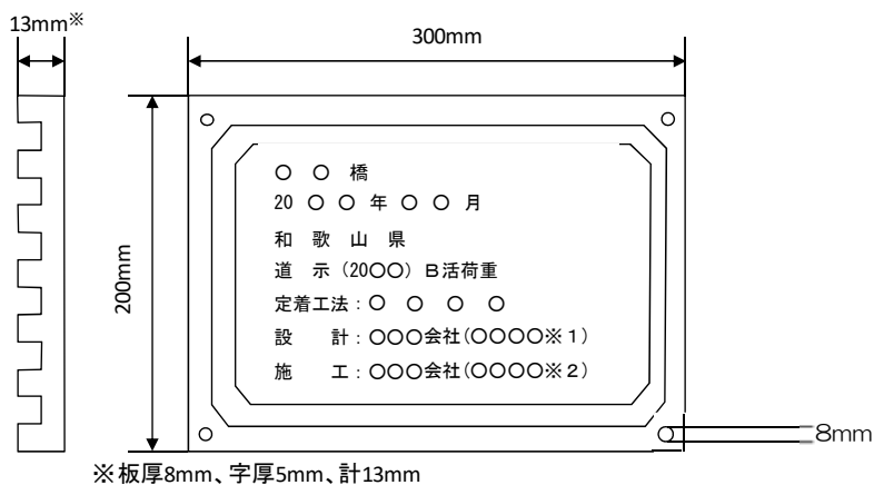
図3-2-2 銘板の寸法及び記載事項
