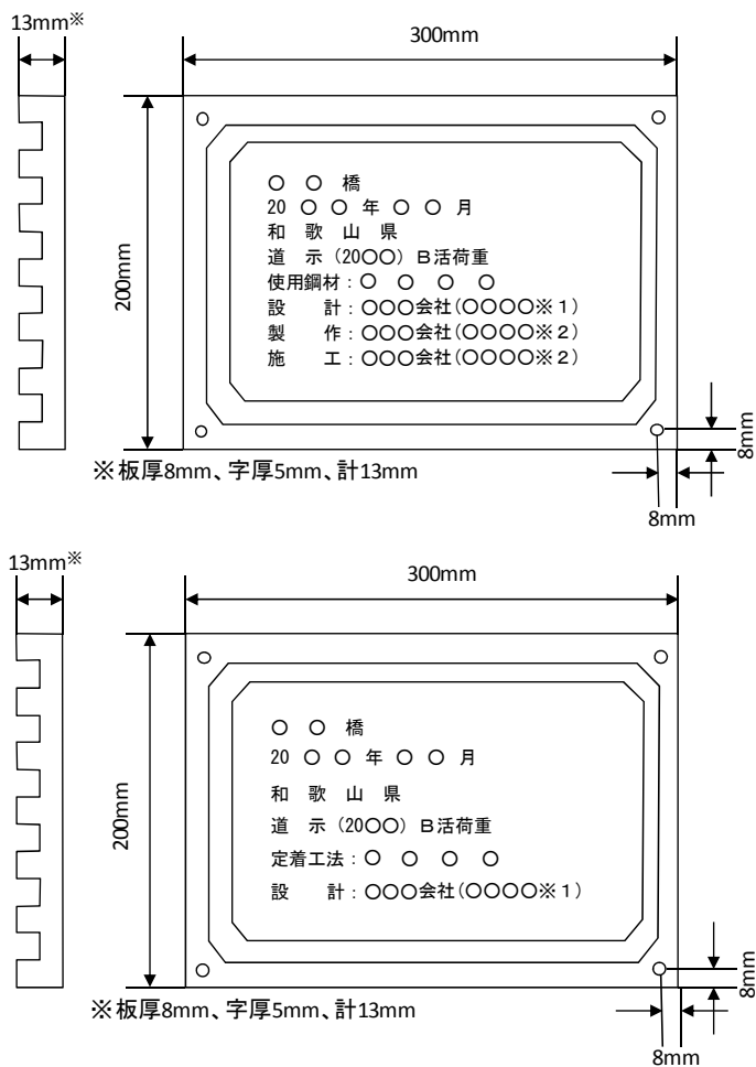
図3-2-2 銘板の寸法及び記載事項
