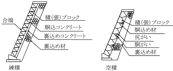
図3-2-5 コンクリートブロック工
