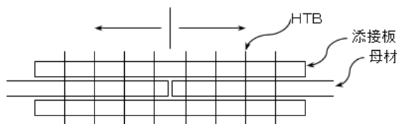
図3-2-1 ボルト締付け順序
