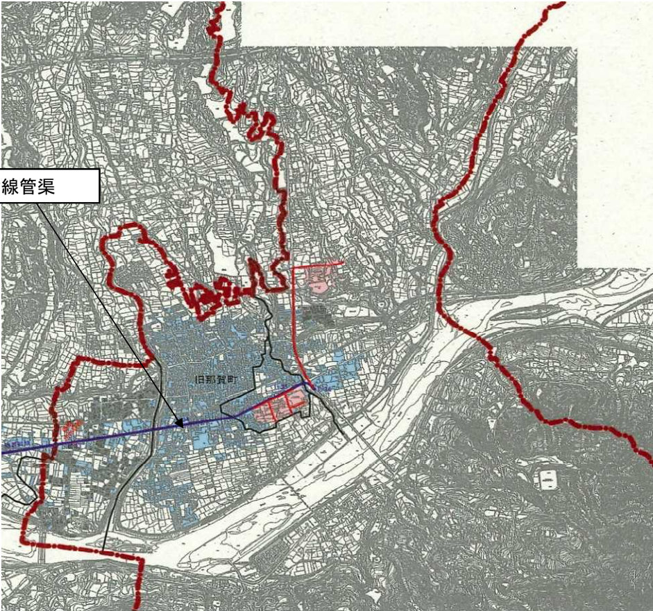
那賀処理区(紀の川市区域)計画図
