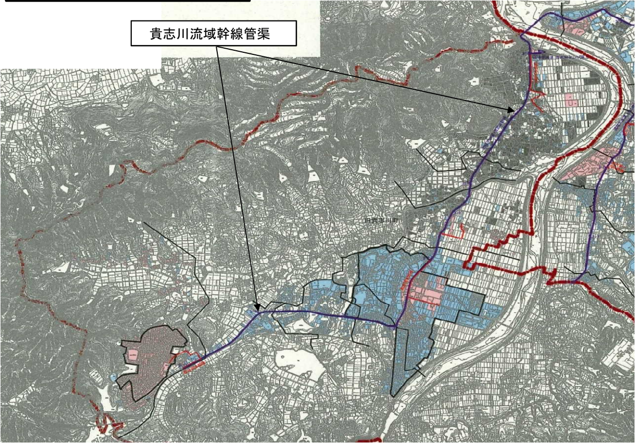
那賀処理区(紀の川市区域)計画図
