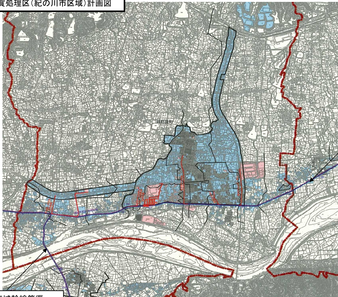
桃山流域幹線管渠
