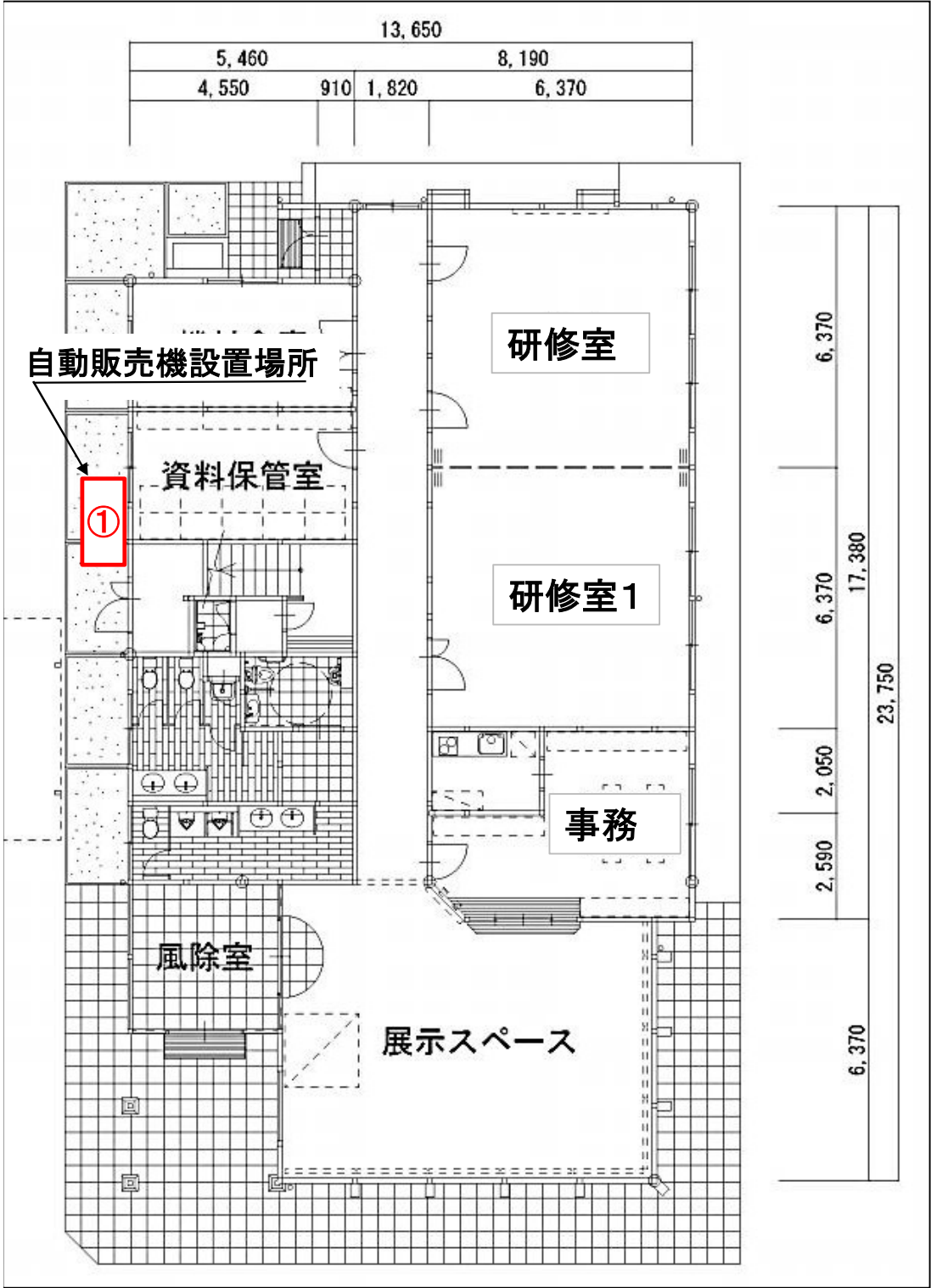
1階平面図
