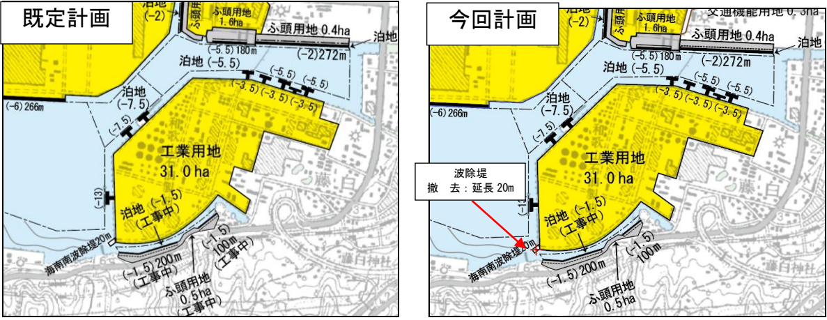
図 2-1-1 海南地区 外郭施設計画（変更箇所）
