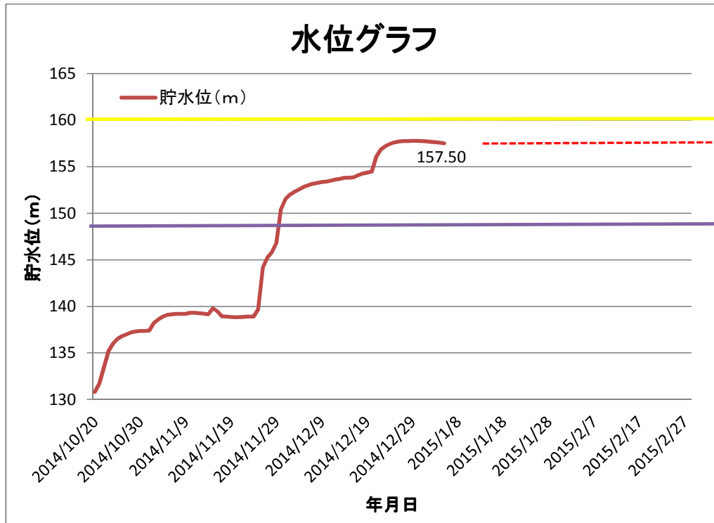
1月5日の湛水状況
