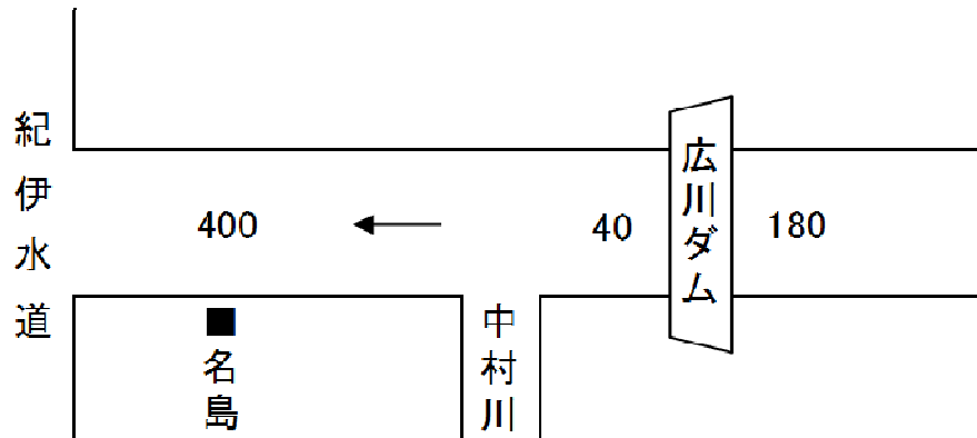
図10 広川水系河川整備計画目標流量配分図
