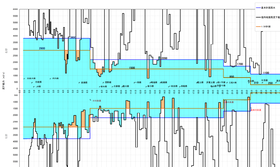
図 2.2 現況流下能力図
