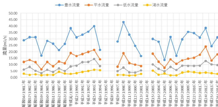
図 2.3 古座川の流況（月野瀬地点）
