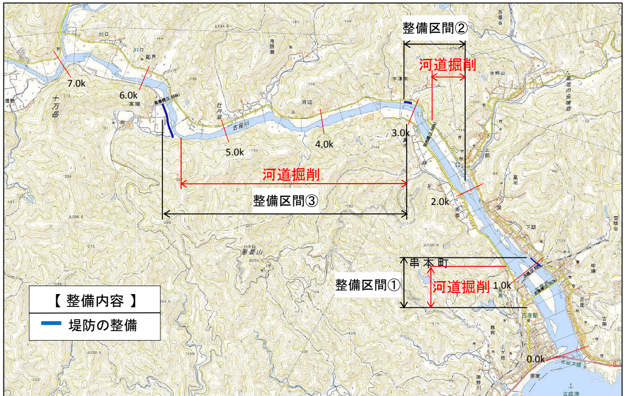
図 4.2 計画的に河川工事を実施する区間
