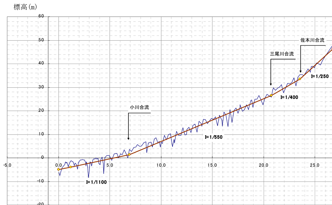
図 1.3 古座川河床縦断面図
