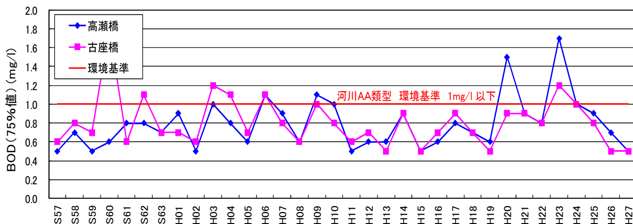
図 2.6 BOD (75%値) の経年変化
