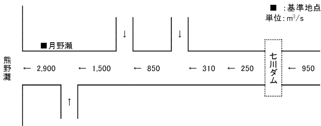
図 4.1 古座川水系河川整備計画目標流量配分図
