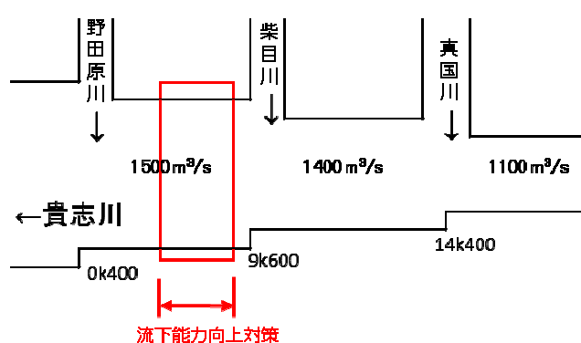
<整備計画流量配分図>
