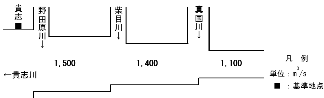
図 4.1 紀の川水系貴志川圏域河川整備計画目標流量配分図
