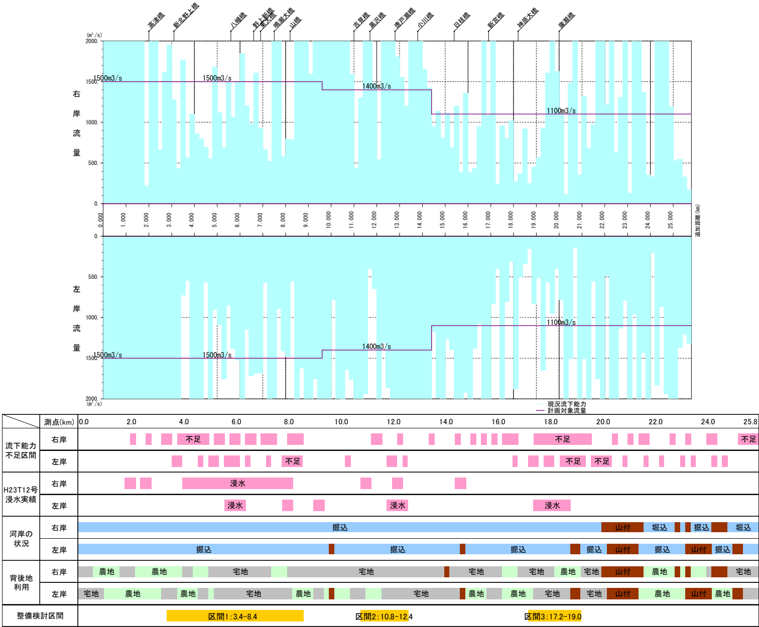
図 2.10 貴志川流下能力図
