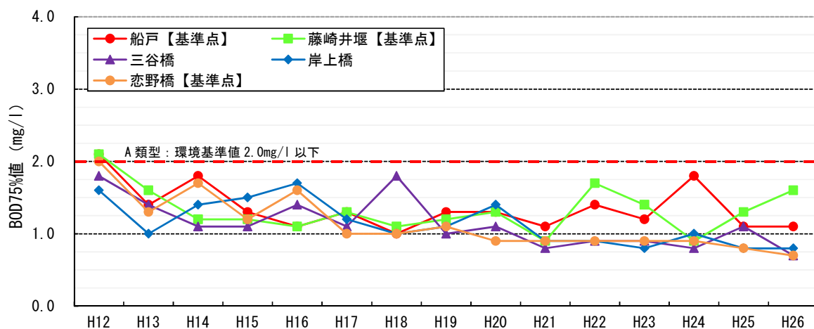
図 2.25 紀の川本川の水質 (BOD75%値)
