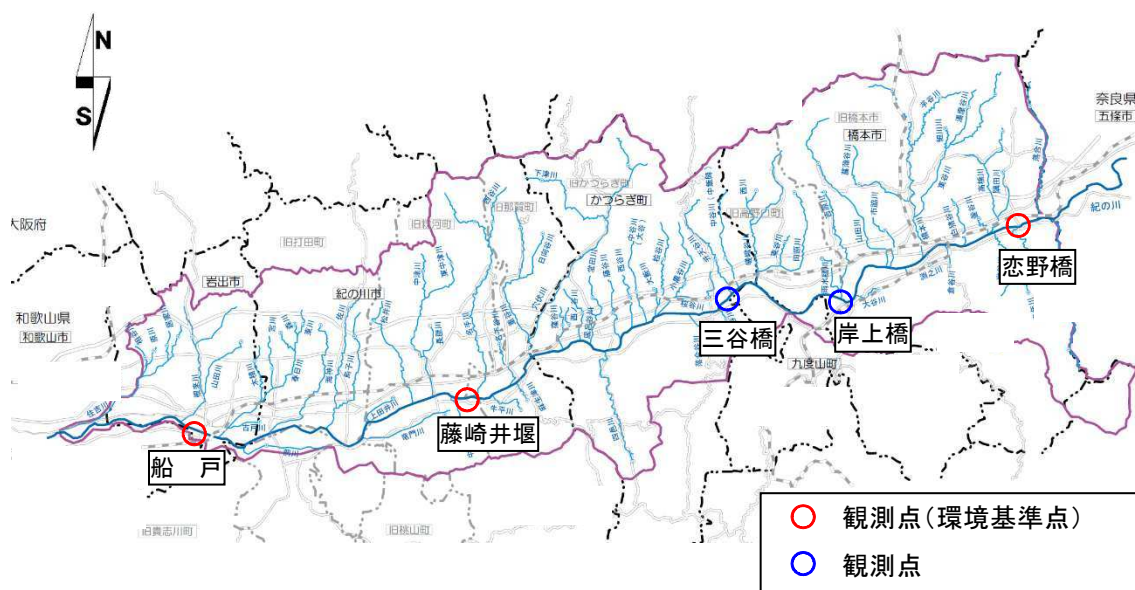
図 2.26 紀の川本川の水質調査地点 (船戸地点上流)
