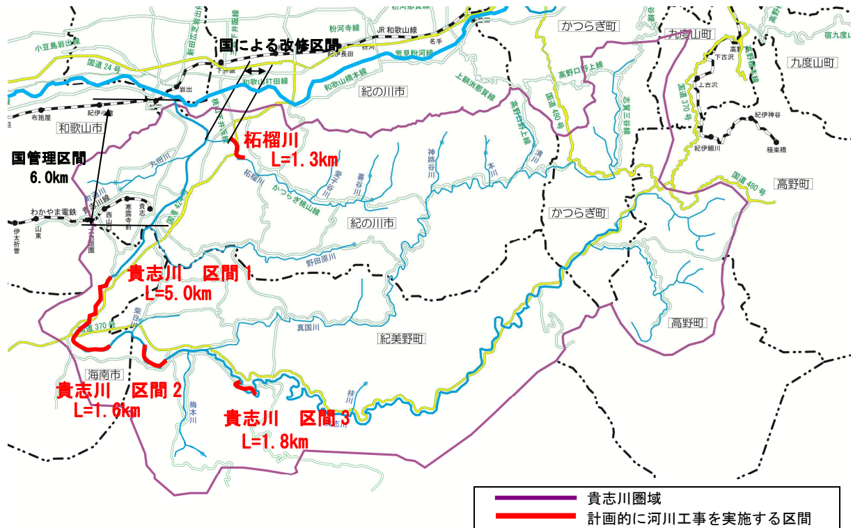
図 4.2 計画的に河川工事を実施する区間
