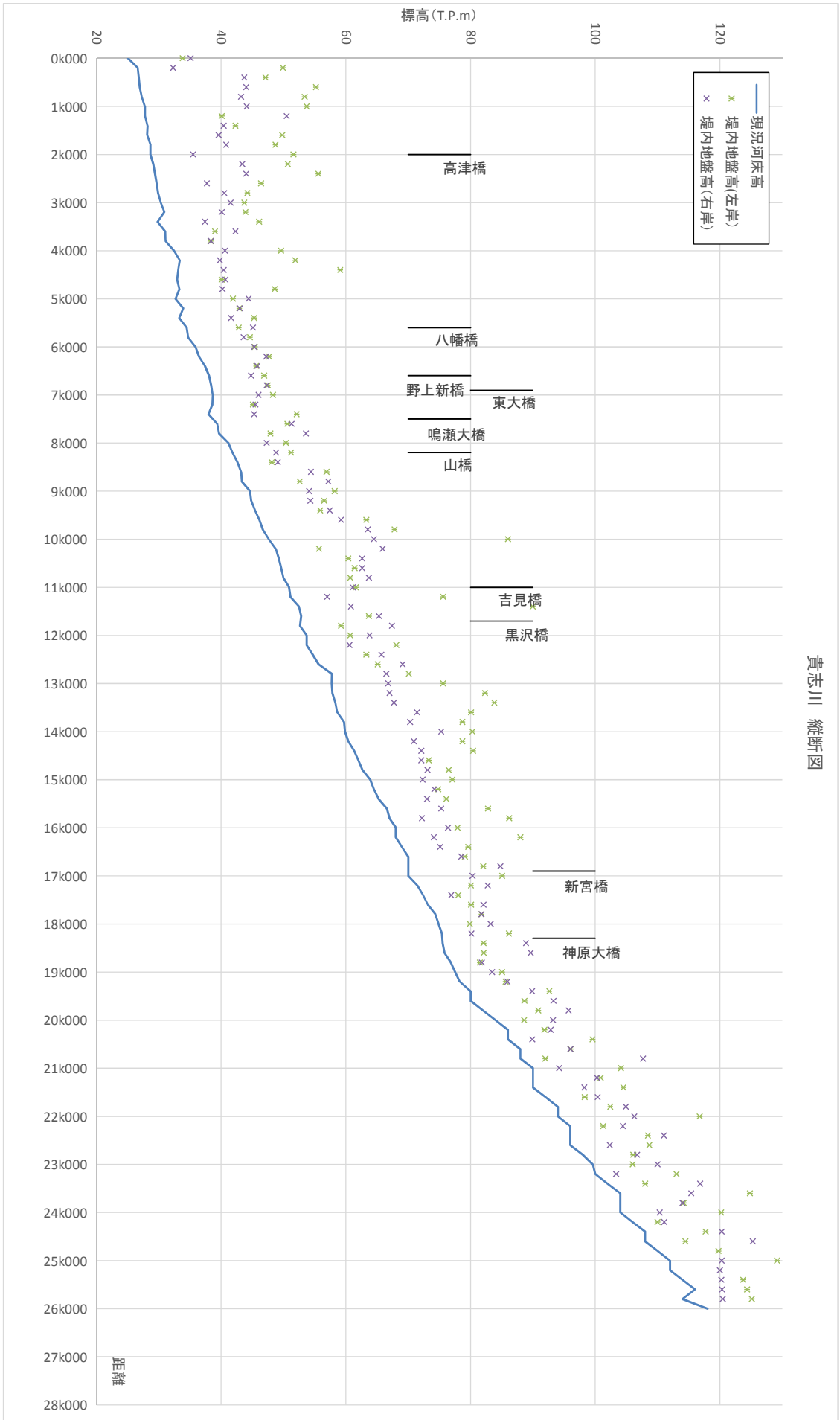
図 2.9 貴志川縦断面図
