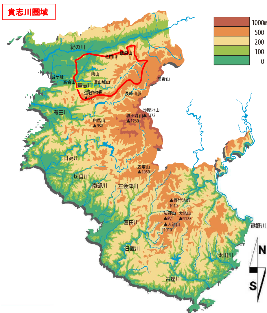
図 1.2 貴志川圏域の地形
