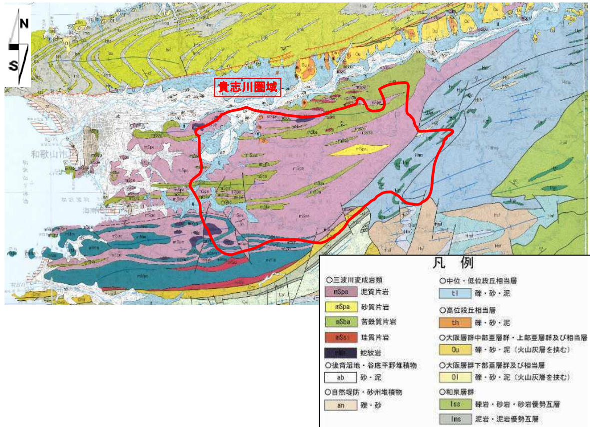
図 1.3 貴志川圏域の地質分類図
