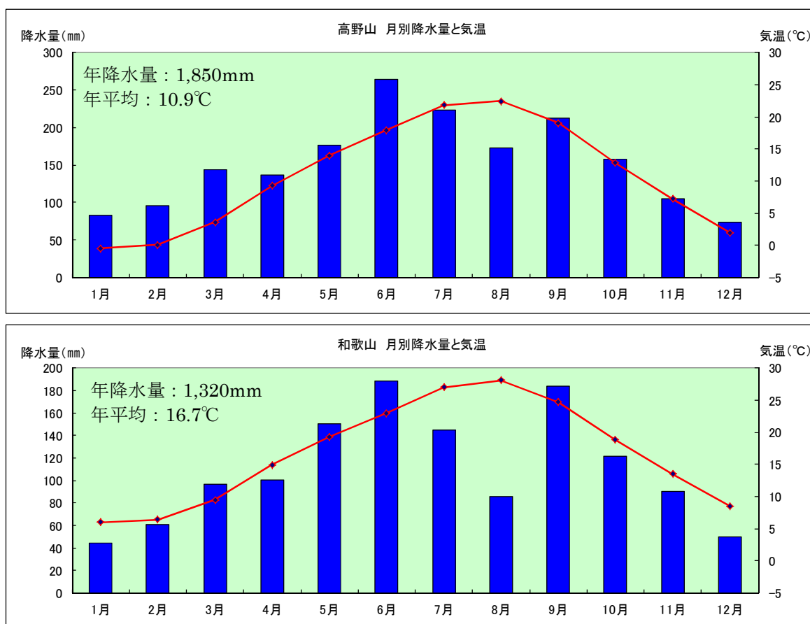
図 1.4 月別降水量と気温
