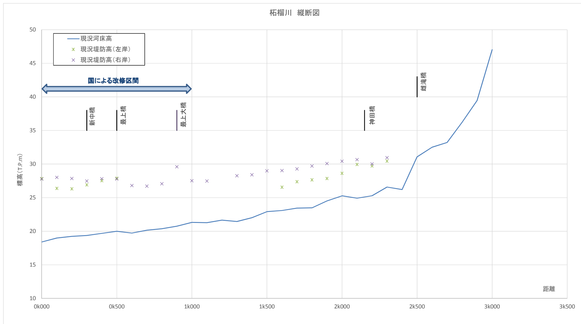
図 2.13 柘榴川縦断面図
