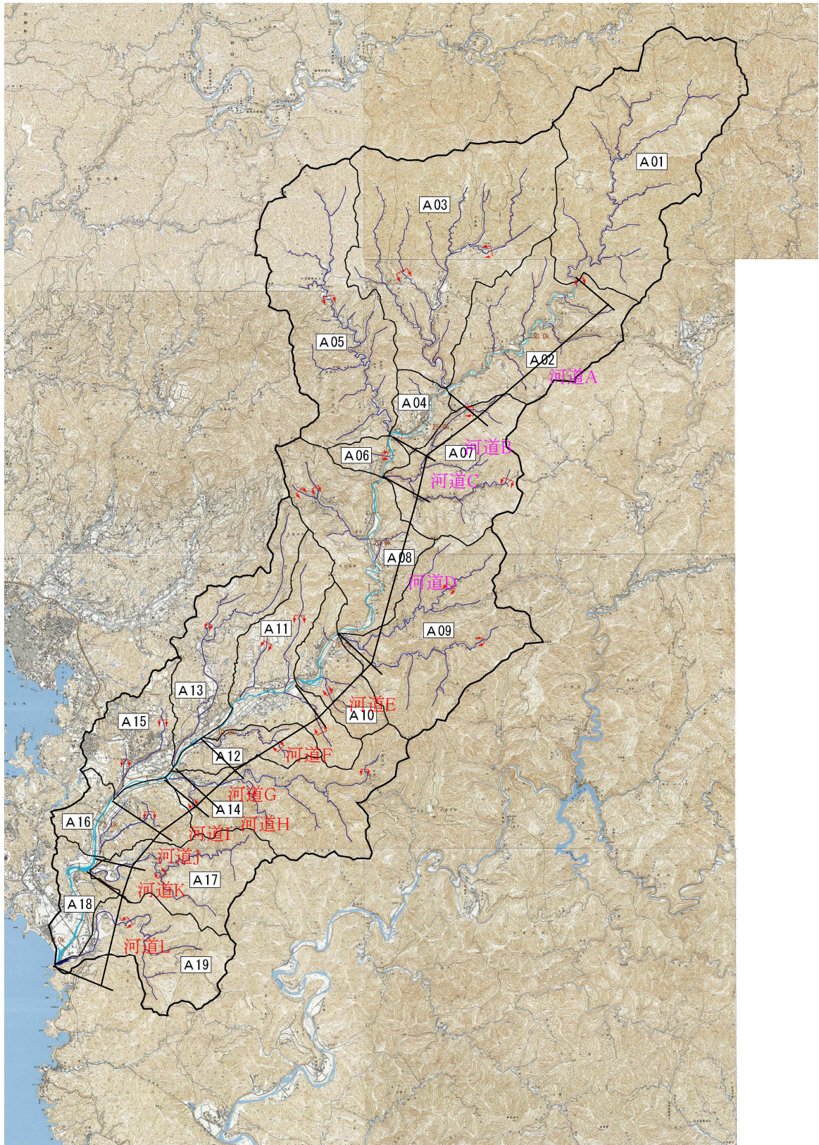
图 2-5-2 流域分割图
