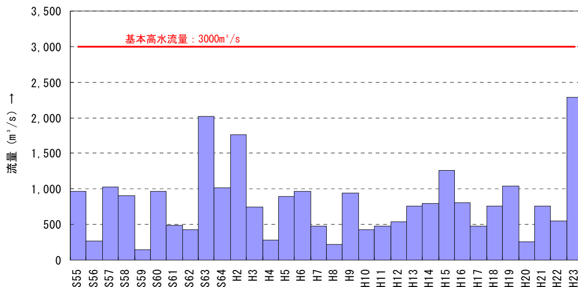
図 2-5-11 庄川口の年最大流量
