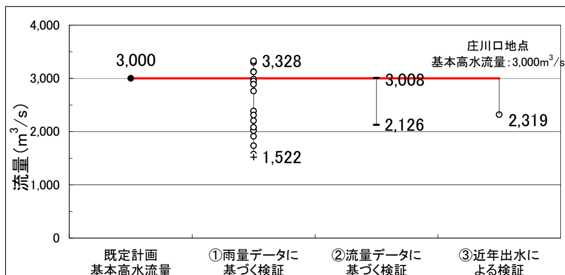
図 2-6-1 各分布による基本高水流量のピーク流量算定結果
