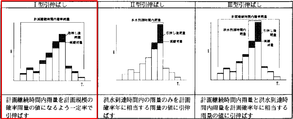
図 2-5-4 Ⅰ型引き伸ばし方法概念図
