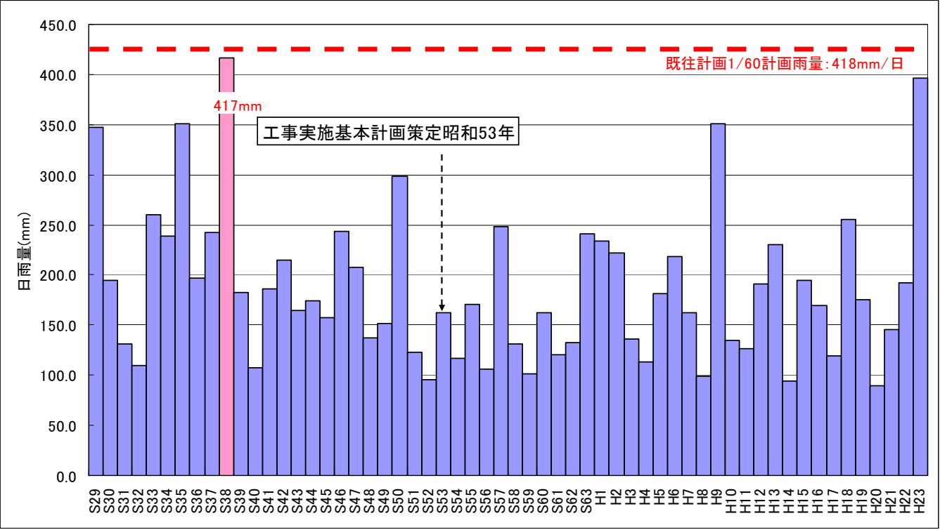
図 2-2-1 年最大日雨量(栗栖川観測所)
