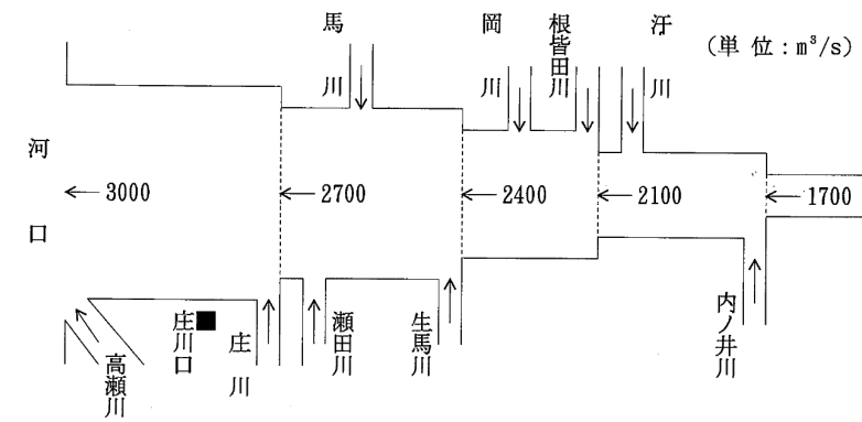
図3-1 計画流量配分図
