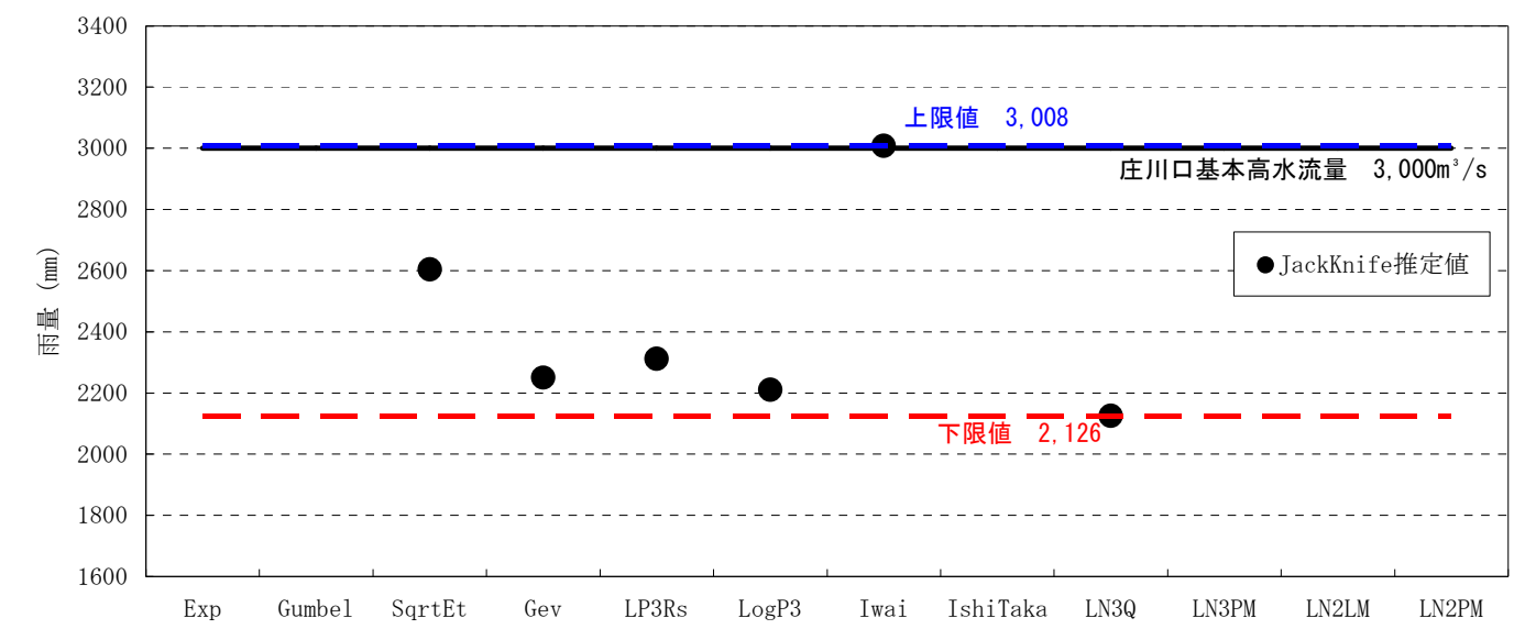
図 2-6-1 庄川口実績流量による確率流量レンジ幅の確認
