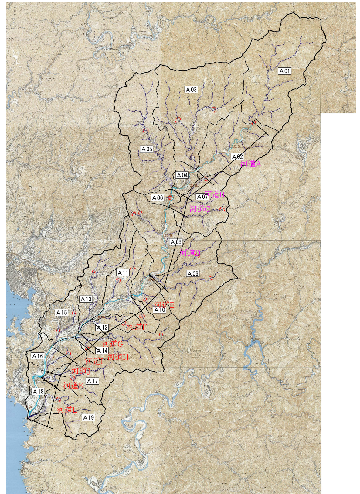
図 2-5-2 流域分割図
