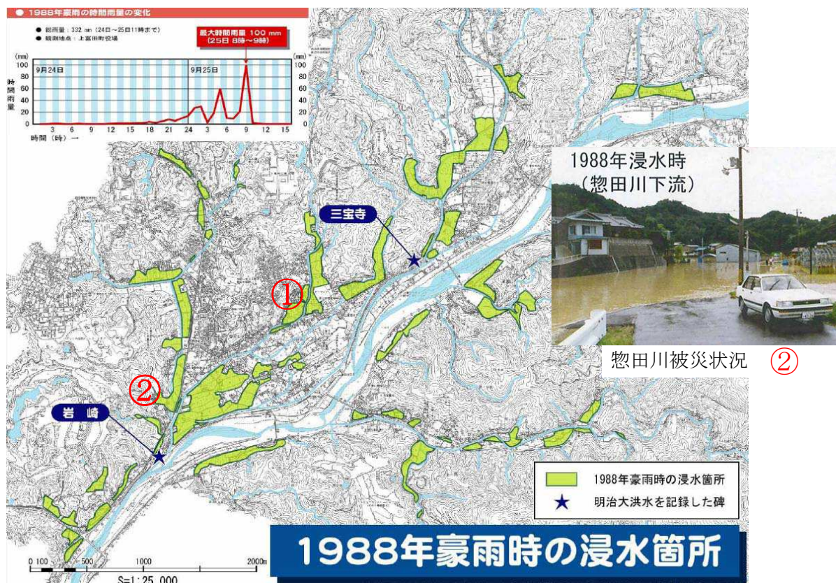
図 1-16 浸水実績位置図 (出典；上富田町洪水ハザードマップ)
