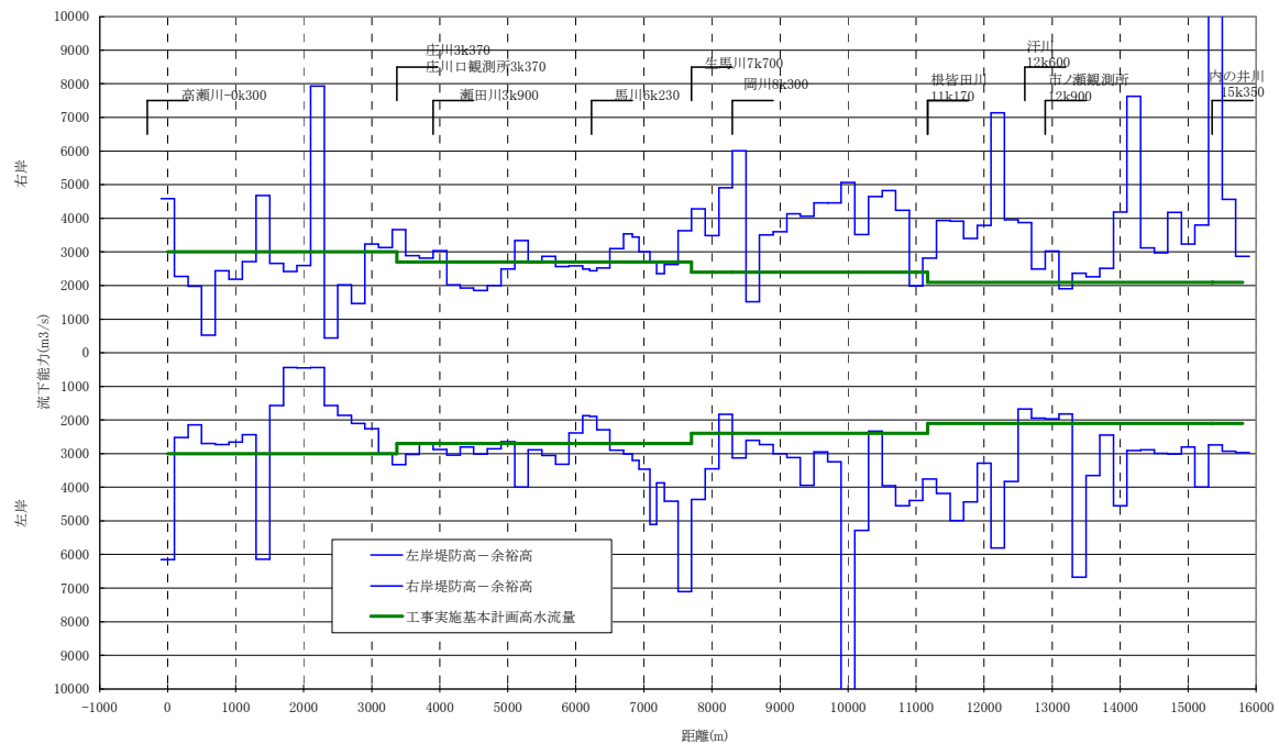
図 1-19 現況流下能力図
