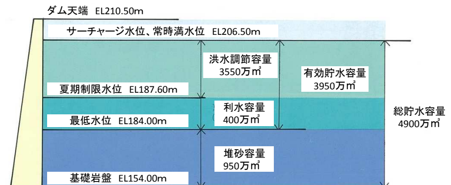
貯水池容量配分図
