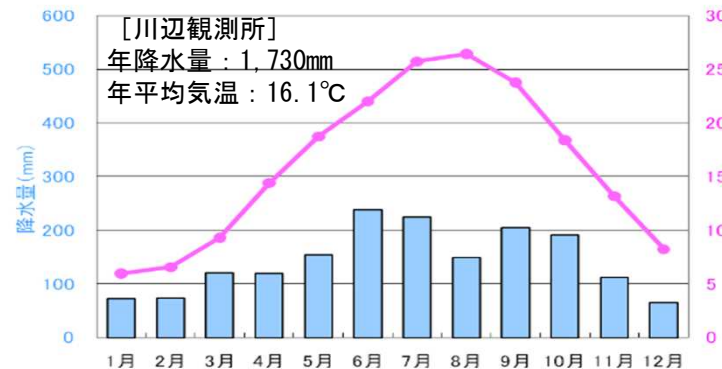
月別降水量と平均気温 (2000年～2009年)
