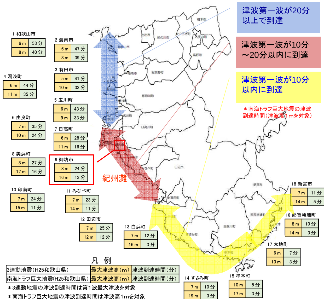
和歌山県で予想されている津波水位と到達時間
