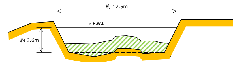
図 6 亀の川改修区間標準横断面図
