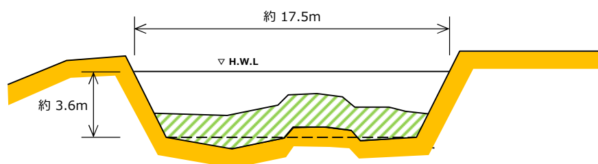
図 6 亀の川改修区間標準断面図
