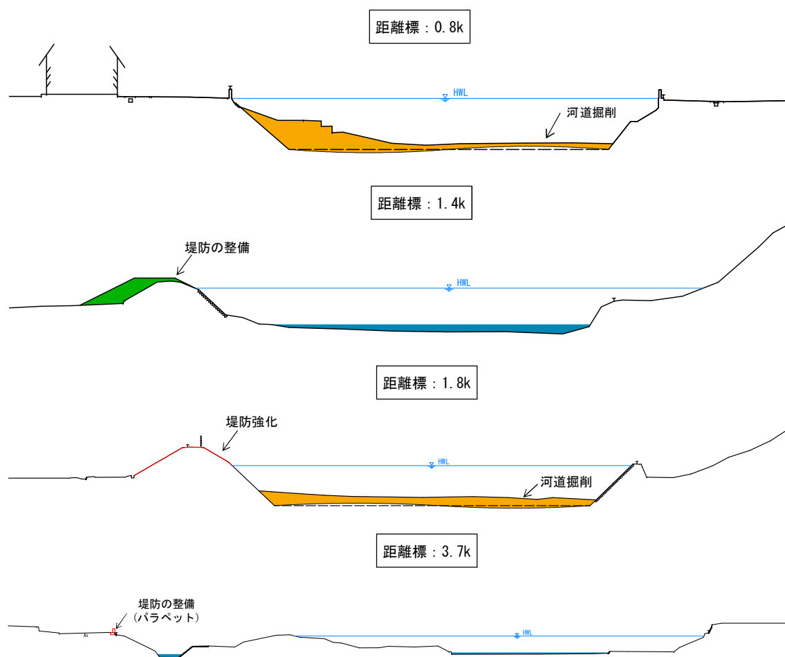
図 4-2 標準断面図
