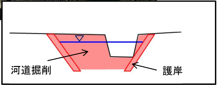
対策イメージ (佐野川)
