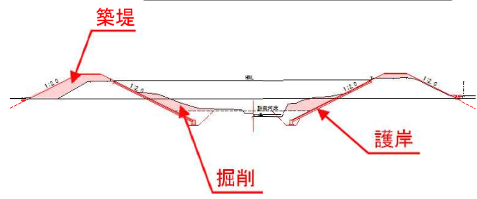
対策イメージ(左会津川)
