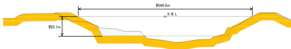
図 5 - 3 標準断面図
