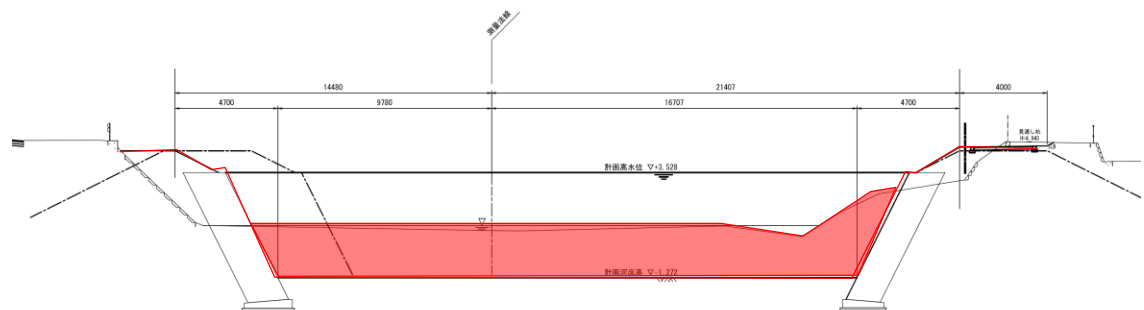
<標準断面図>
