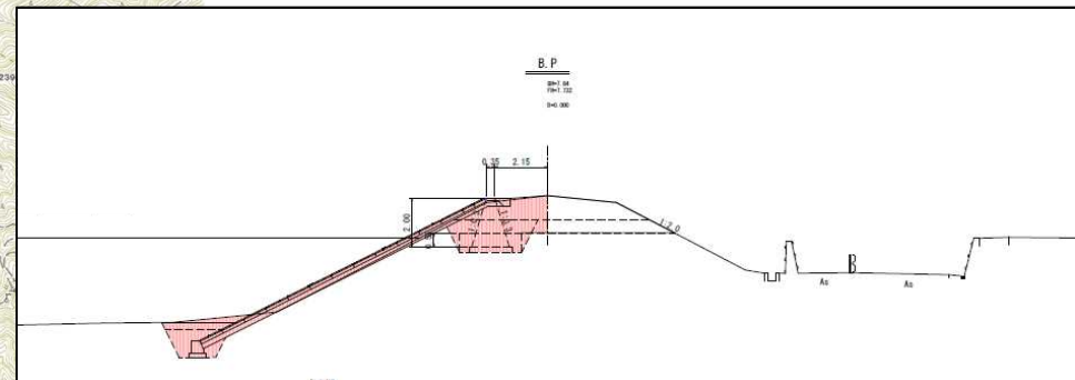
＜標準断面図＞
