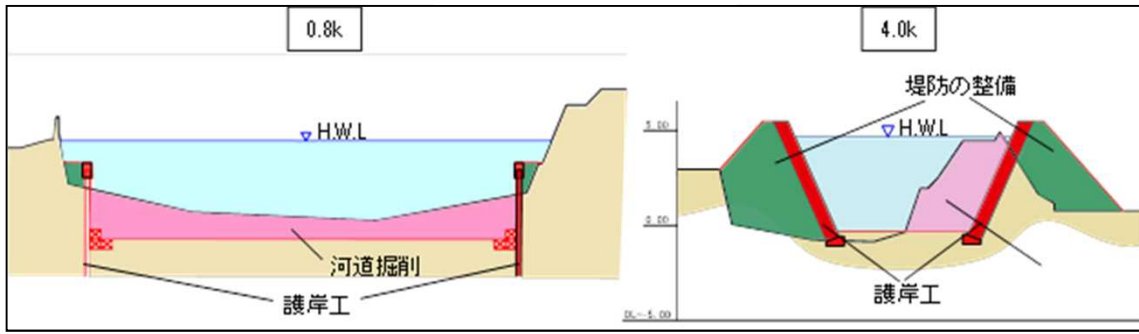
<標準断面図>
