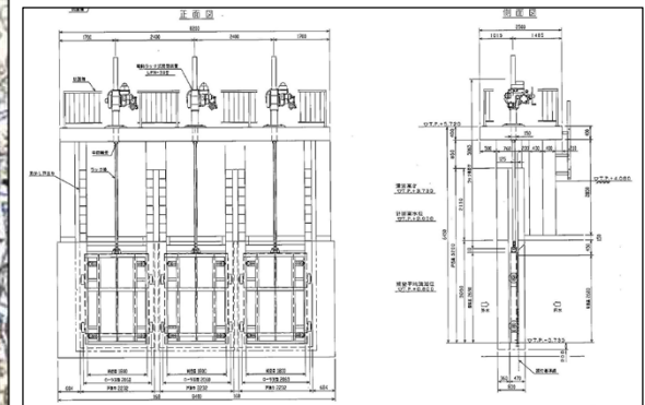
<構造図>
