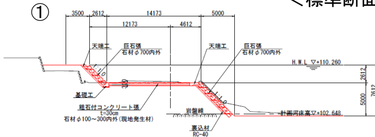
<標準断面図>
