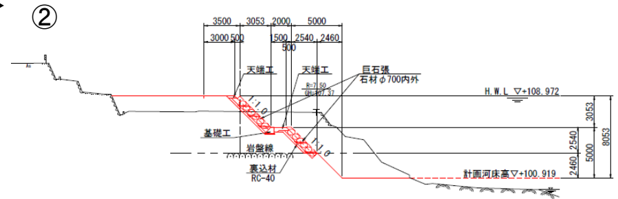
<標準断面図>
