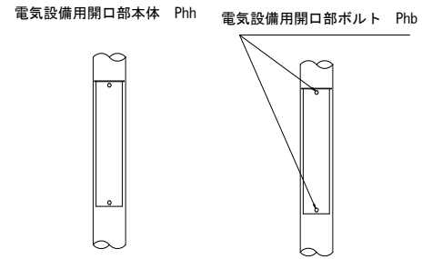
図-解 8-3 主な点検箇所（各形式共通 支柱基部および電気設備用開口部）
