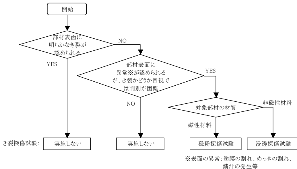
図-解 8-14 き裂探傷試験実施の目安
