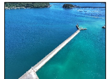
防波堤の改良（串本漁港）
