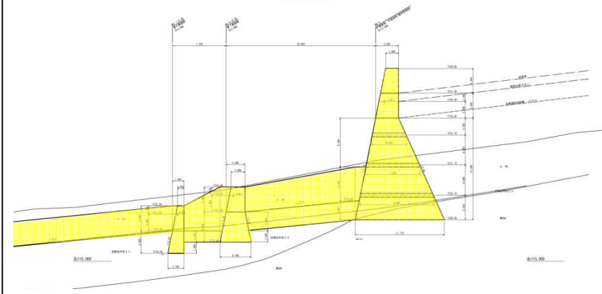
砂防えん堤工側面図
