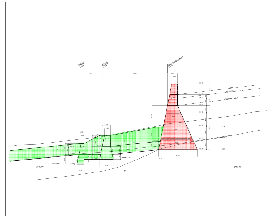
砂防えん堤工側面図
