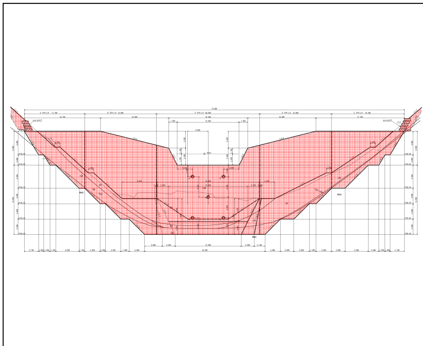
砂防えん堤工正面図
