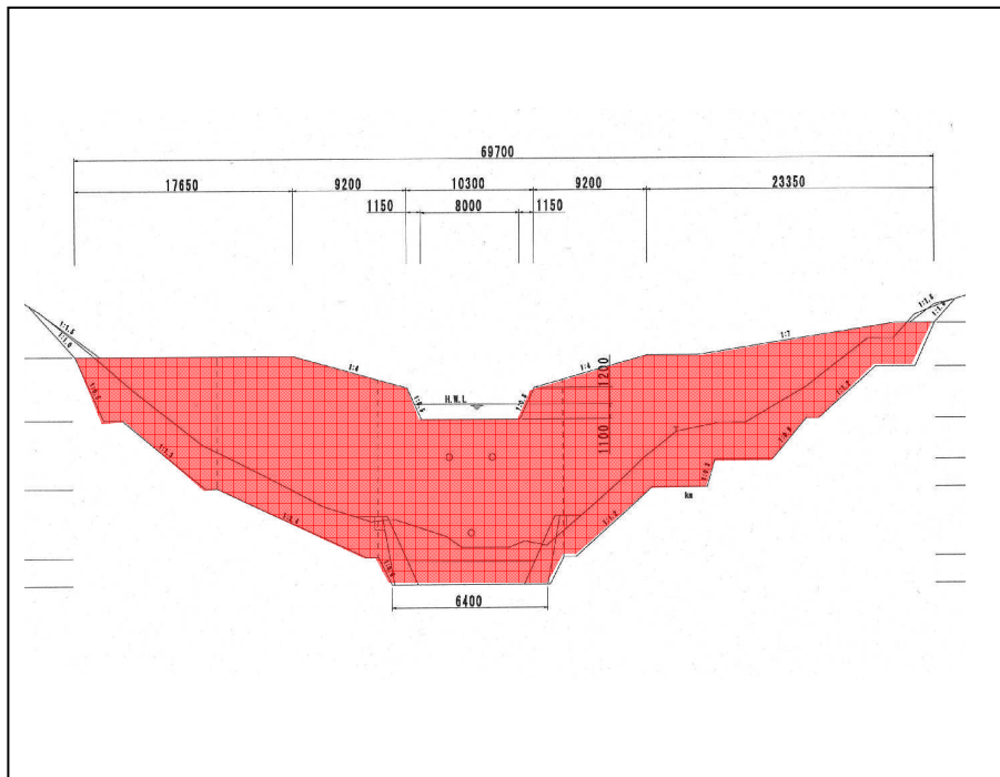
砂防えん堤工正面図
