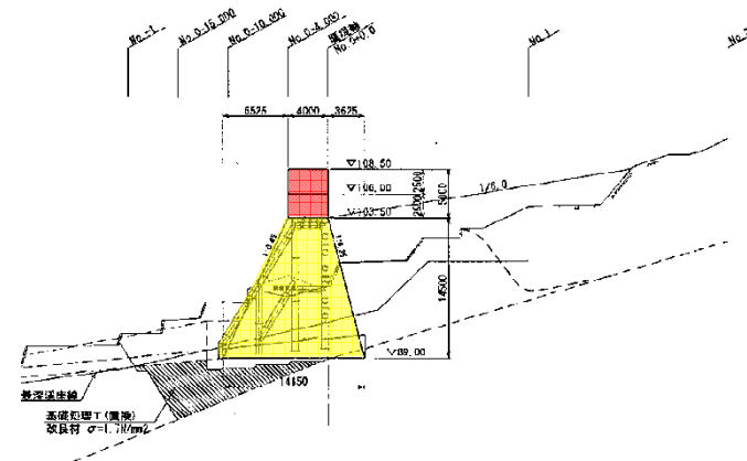
砂防えん堤工側面図
