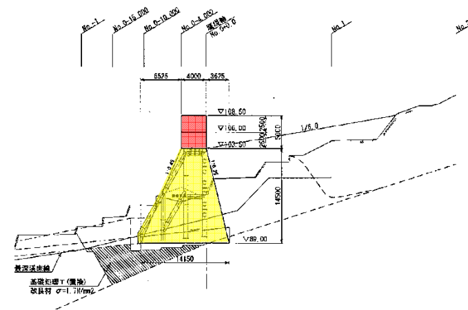
砂防えん堤工側面図
