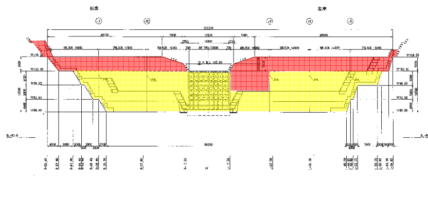
砂防えん堤工正面図
