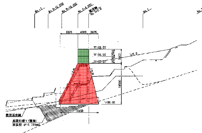
砂防えん堤工側面図
