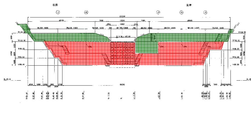
砂防えん堤工正面図
