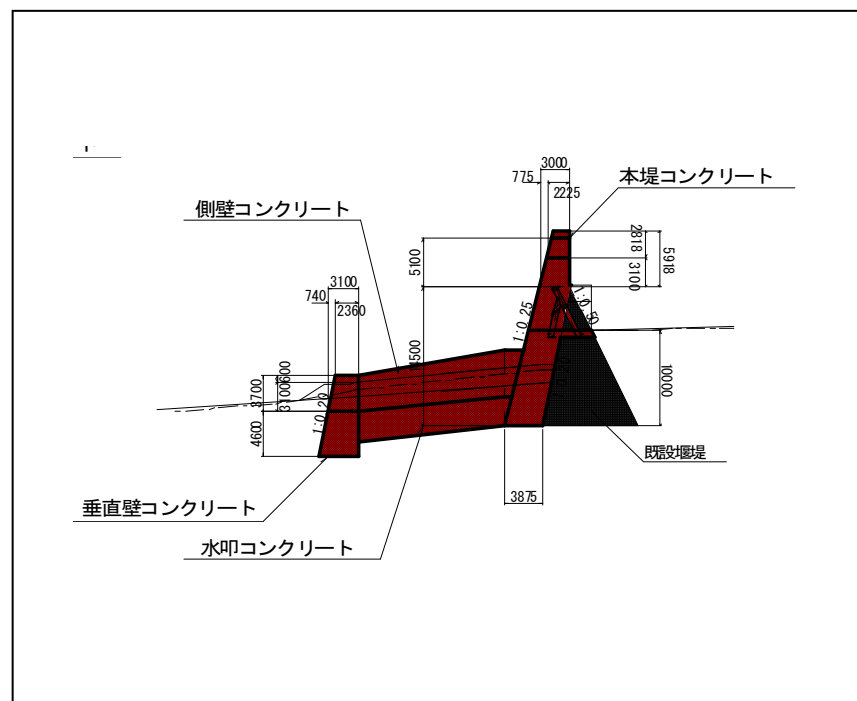
2号砂防えん堤側面図
