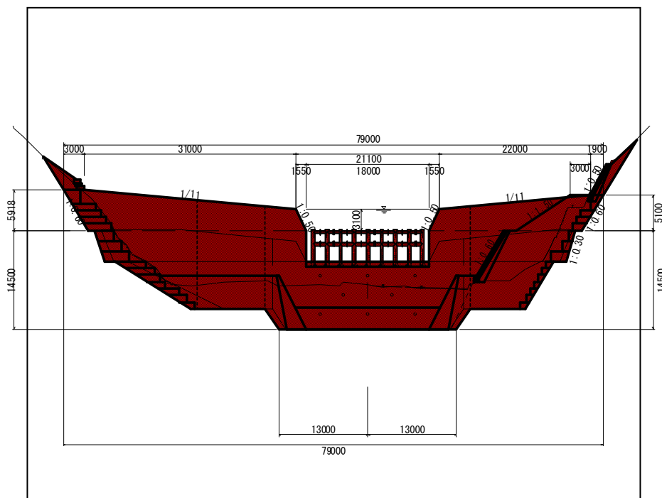
2号砂防えん堤正面図
