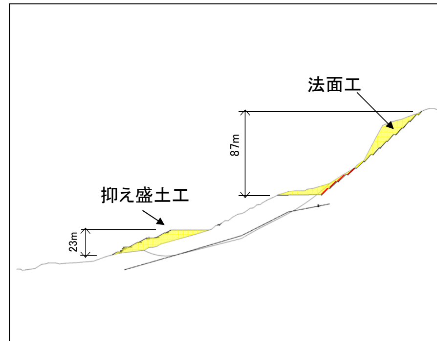
断面図
