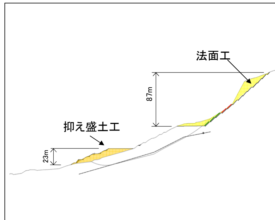
断面図
