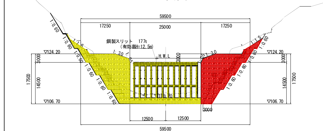
正面図
