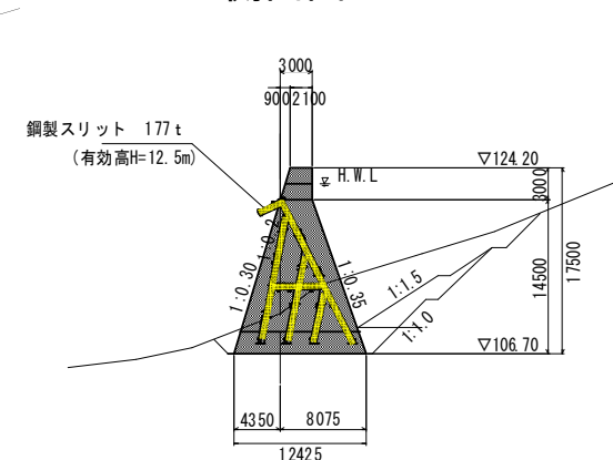
側面図
