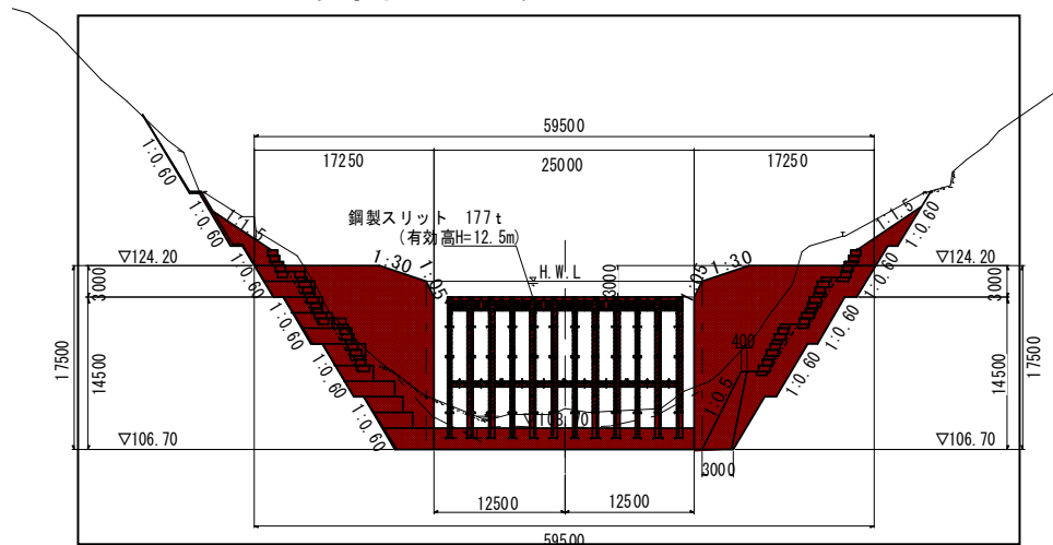
砂防えん堤工正面図
