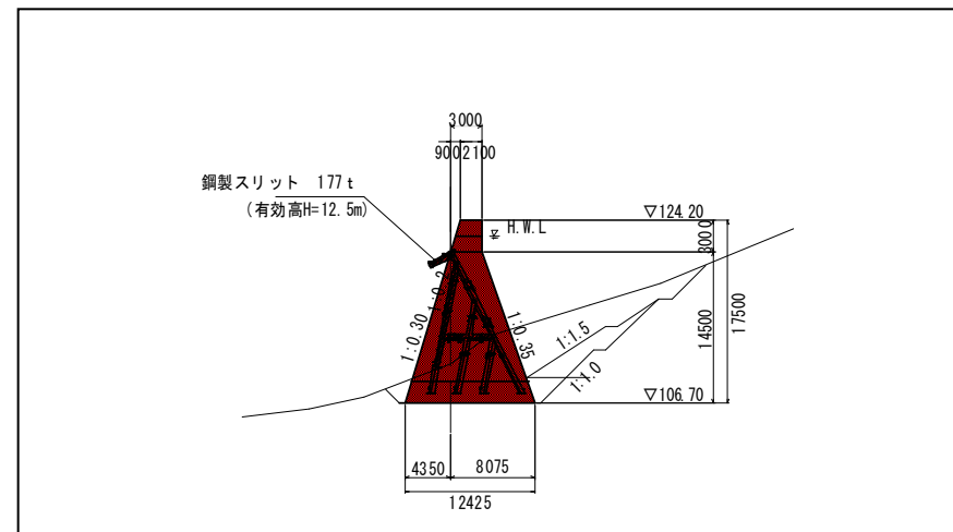
砂防えん堤工側面図
